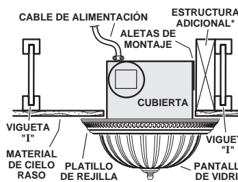
CUBIERTA MONTADA EN UNA VIGUETA "1" Se requiere una estructura adicional para las aletas de montaje. Descarga paralela a las viguetas.
