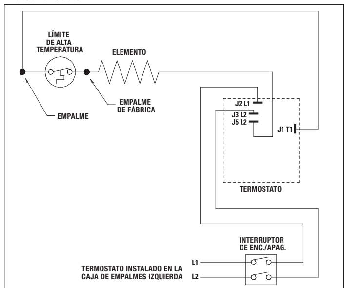
FIGURA "B" (cableado de la caja de empalmes derecha)
