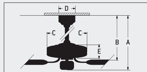
A: 6" DR - 16.25" B: 6" DR - 13.25" C: 13.5" D: 6" E: 5" *DR=Downrod
