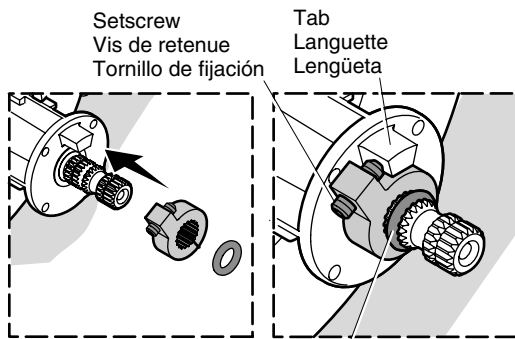
O-Ring/Joint torique/Arosello
