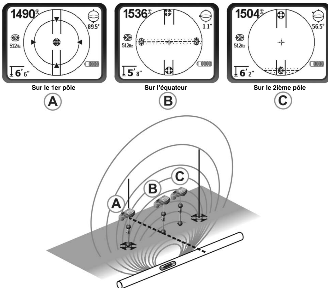
Figure 24 – Affichages obtenus à différents endroits (mode « Sonde »)
