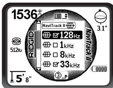
Figura 18 – Las frecuencias seleccionadas aparecen marcadas
