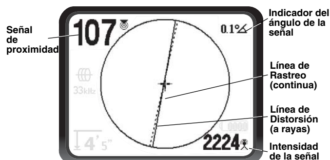
Figura 8 – Elementos en el display de Modalidad 'Rastreo de Conductos Activados'
