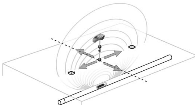
Figura 22 – Polos y Ecuador de una Sonda
