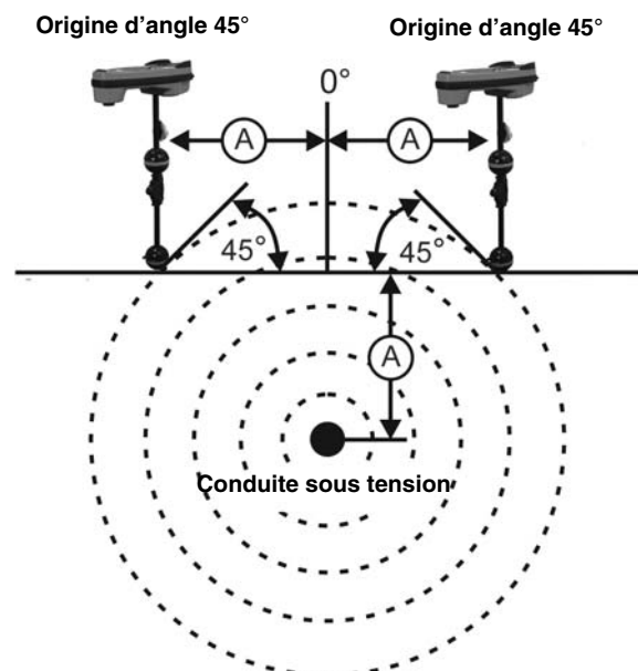
Figure 30 – Dépistage des distorsions
