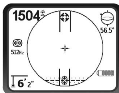
Aproximándose al segundo Polo
