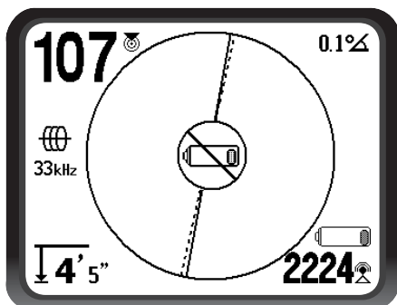
Figure 10 – Affichage de l'avertissement « piles déchargées »
