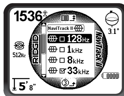
Figura 16 – Realce de la frecuencia deseada (128 Hz)
