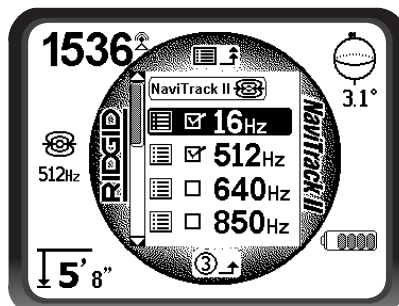
Figure 44 – Sélection d'une fréquence à activer
