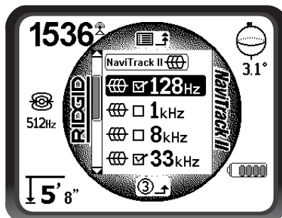
Figure 18 – Fréquence voulue cochée
