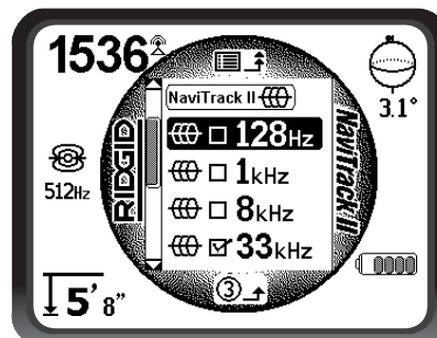
Figure 16 – Fréquence voulue (128 Hz) surlignée
