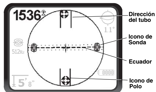
Figura 7 – Elementos en el display de Modalidad 'Sonda'
