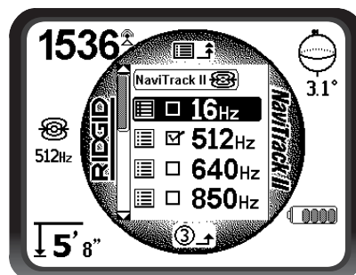
Figura 44 – Selección de una frecuencia para activarla
