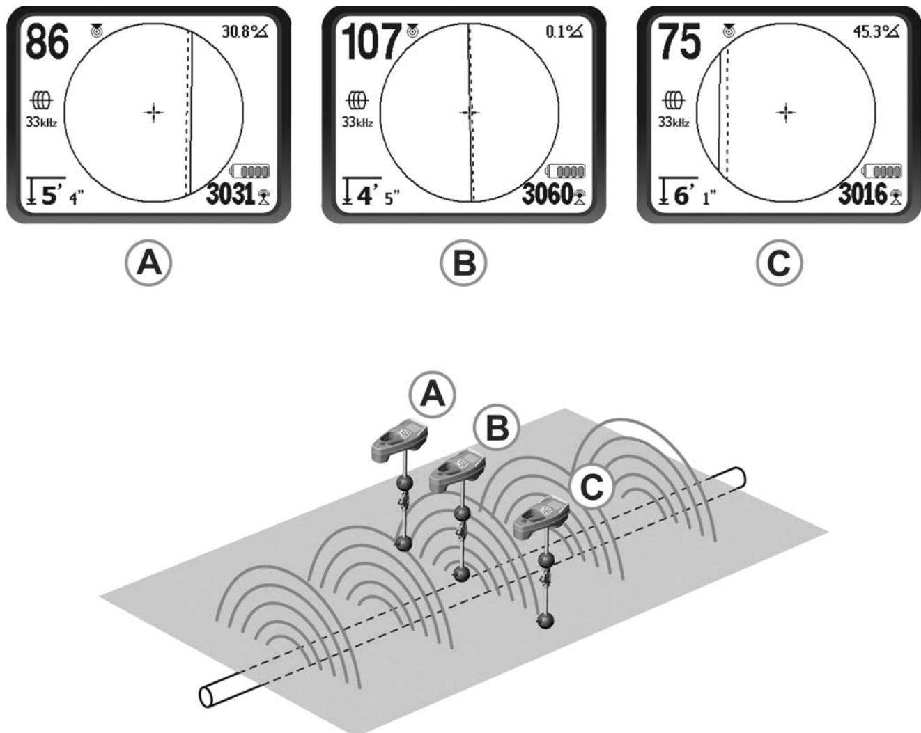
Figura 28 – Lo que aparece en pantalla cuando el NaviTrack II se sitúa en distintas posiciones (Rastreo de Conductos Activados)
