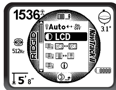
Figura 34 – Opciones de contraste
