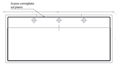
Vista zenitale
