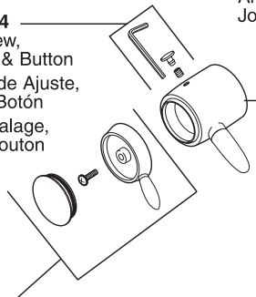
RP53415▲ Temperature Knob, Cover & Screw Perilla de la Temperatura, Cubierta y Tornillo Poigné de Réglage de Température et Vis
