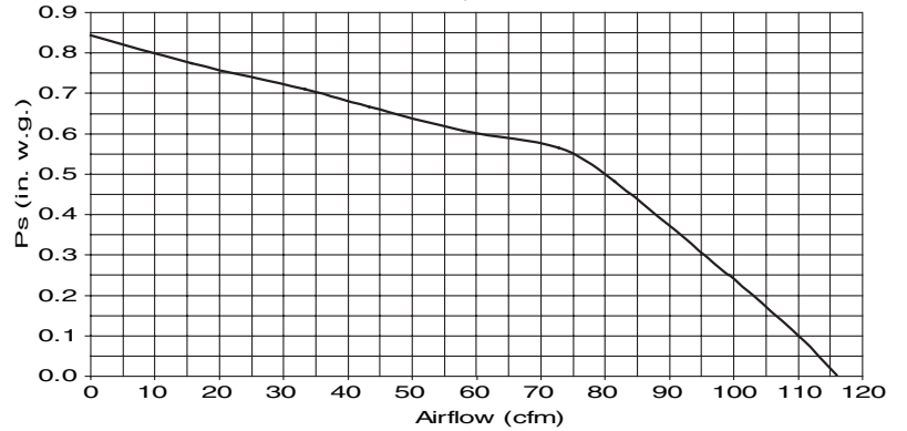
MODEL QTR110L
