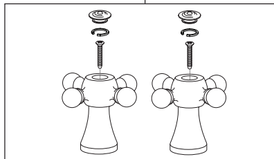
RP52400▲ Cross Handle w/Button, Friction Ring & Set Screw Manija con Botón, Arandela de Fricción y Tornillo de Ajuste Manette avec Bouton, Rondelle de Friction et Vis de Calage
