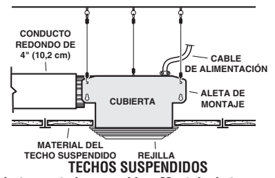
Cubierta montada con cables. Montaje de tres puntos.
