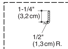
Detalle del reborde integral
