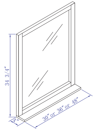
ME/MW3034MR ME/MW3634MR ME/MW4834MR
