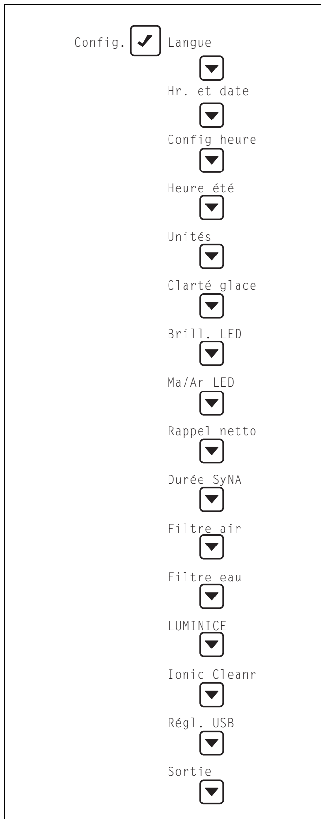
Menu Config
